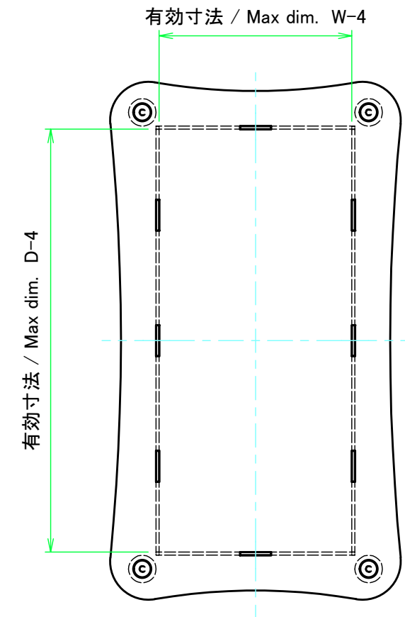
下カバー / Bottom cover
